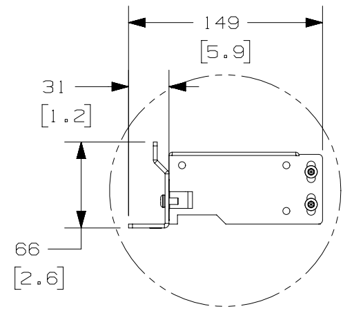
DETAIL B SCALE 1 : 4 TYP - LEFT & RIGHT
